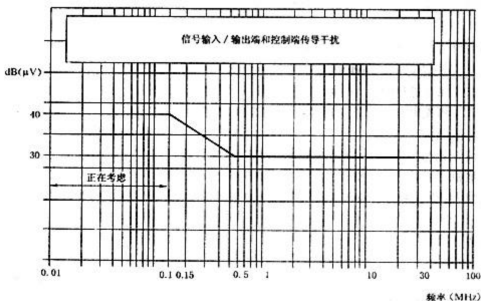
图 4 传导发射的限值(信号输入/输出端和控制器)
