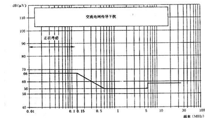
图 3 传导发射的限值(交流输入端)
