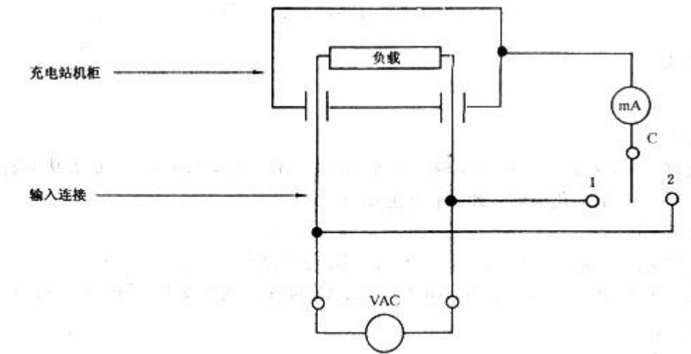
图 1 I 级单相设备漏电流的测量原理图
